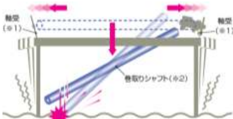
(※1) 軸受：胴体に固定し巻取りシャフトを保持するもの。 (※2) 巻取りシャフト：シャッターカーチンを巻き取る軸。
