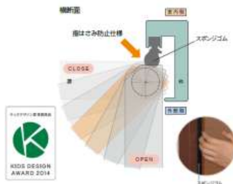
マンションドア指はさみ防止仕様
