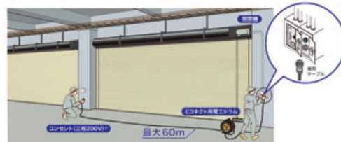
シャッター開放用電源供給システム「Eコネク」
