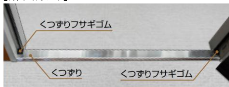
【扉開放時】
